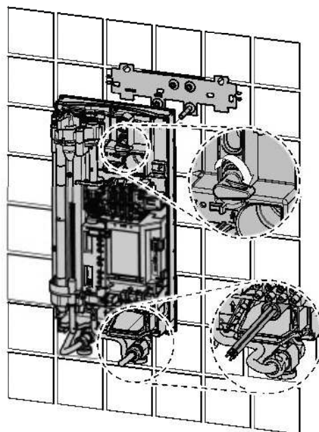
Подвешивание прибора
