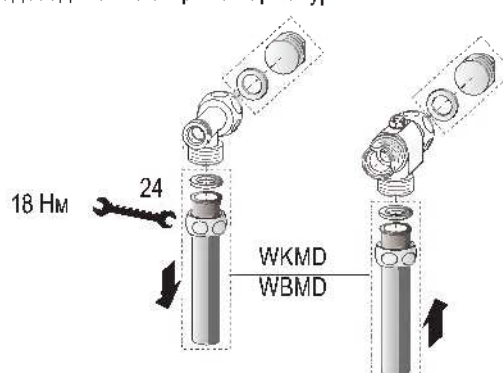
Подсоединение открытой арматуры
