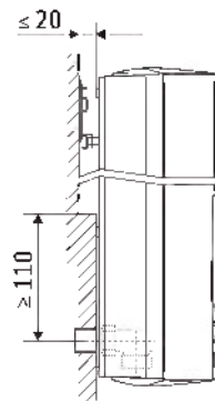
Монтажные размеры при смещении облицовочной плитки
