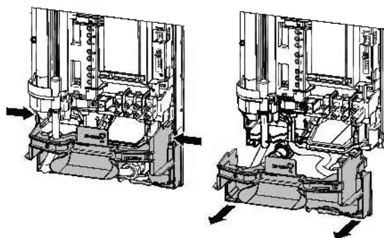
Съем нижней части задней панели
