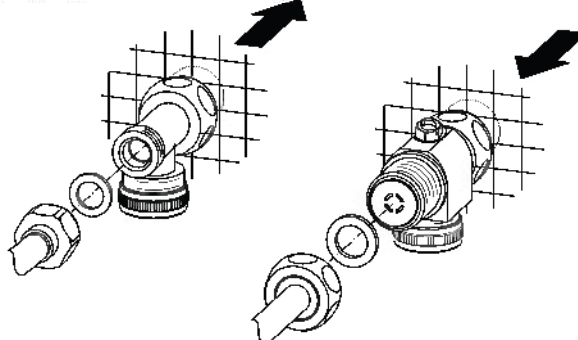
Подвод воды
