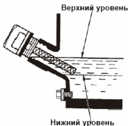
Крышка маслозаливной горловины /щуп
