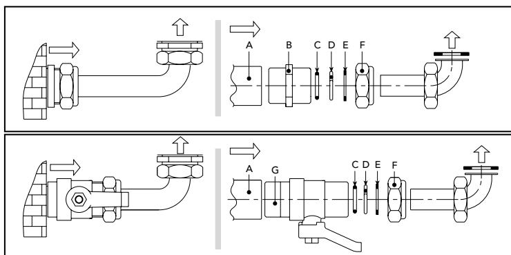
рис. 7 - Соединительный комплект
