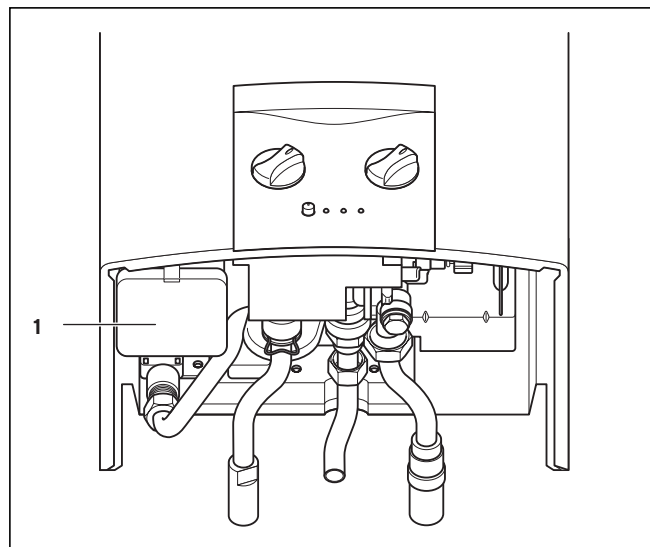
Рис. 4.9 Замена батарей
