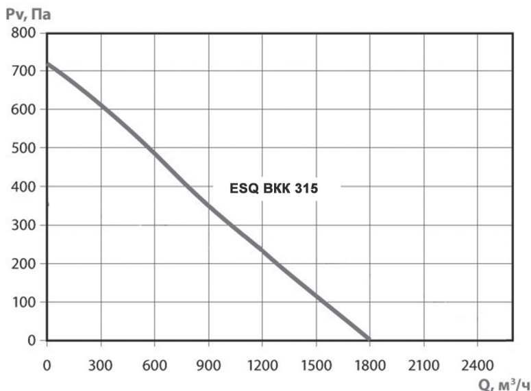
Аэродинамическая характеристика вентилятора ESQ BKK 315.
