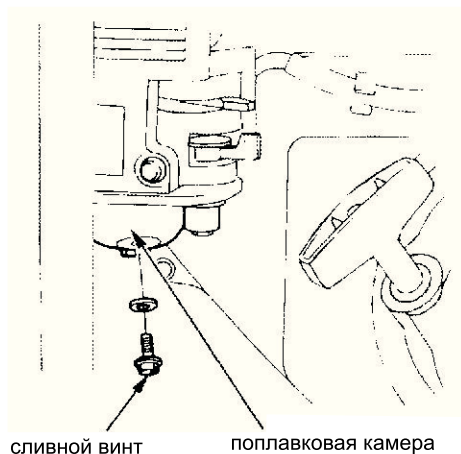
сливной винт
