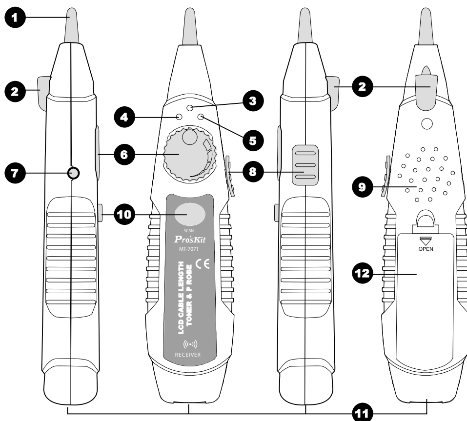
Рис. 2. Схема приемника MT-7071
