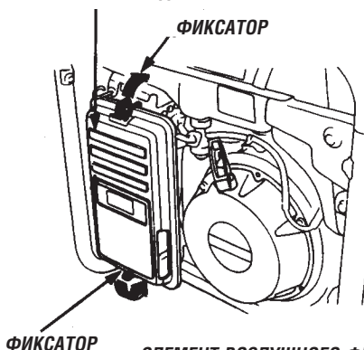
ЭЛЕМЕНТ ВОЗДУШНОГО ФИЛЬТРА
