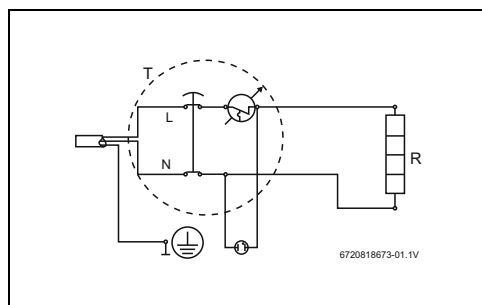
Рис. 6 Схема соединений
