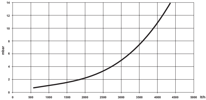
рис. 11 - Гидравлическое сопротивление системы
