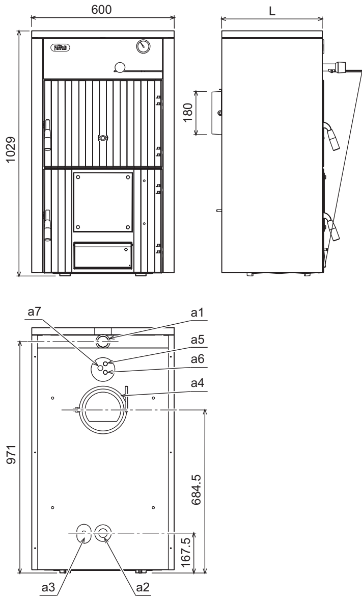
рис. 10 - Габаритные размеры и присоединения
