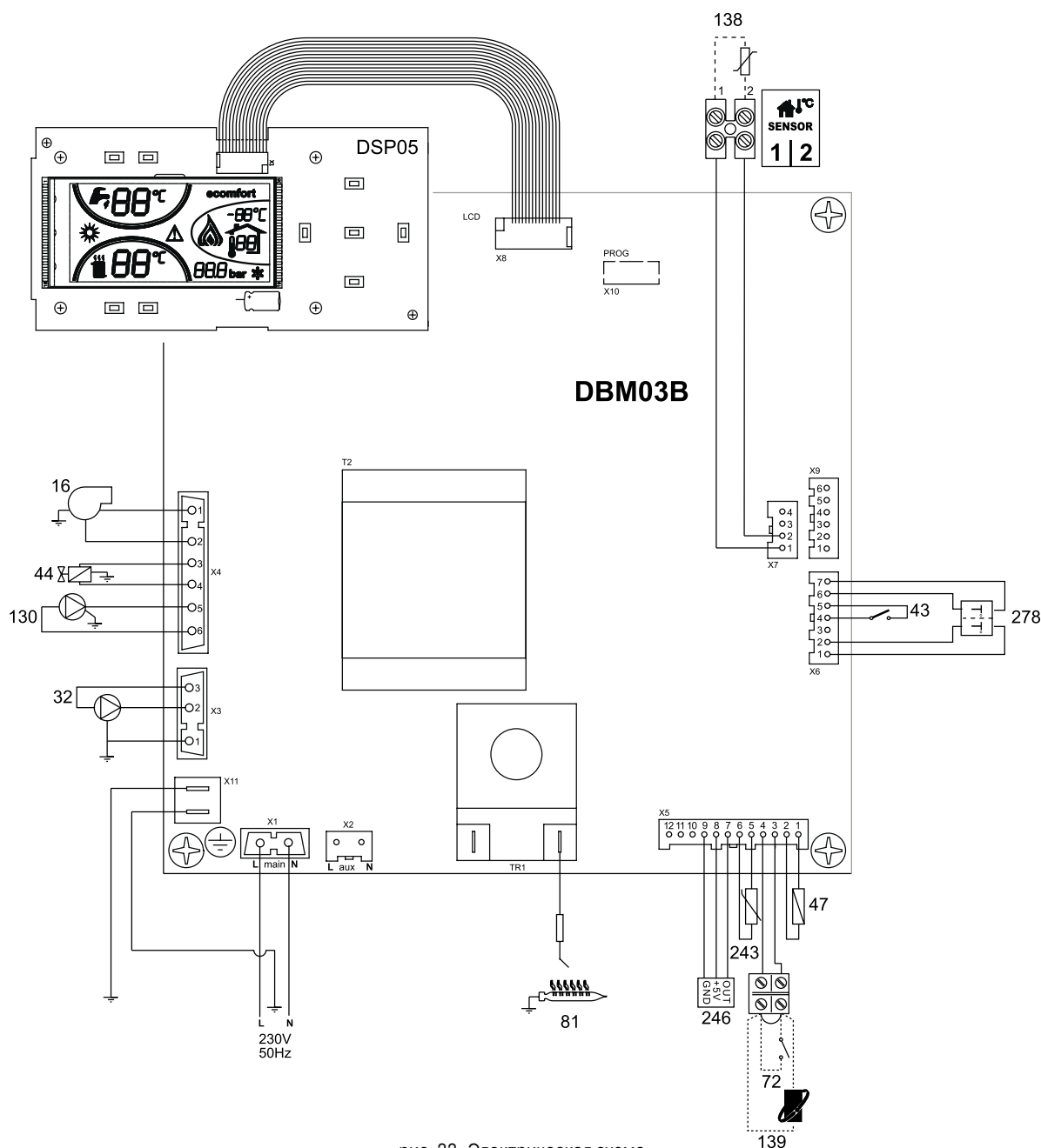
рис. 33 -Электрическая схема
