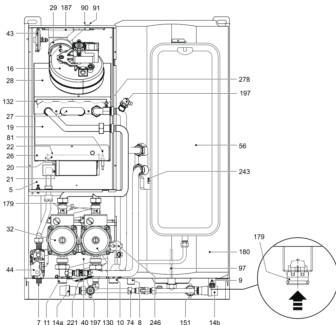
рис. 31 - Общий вид
