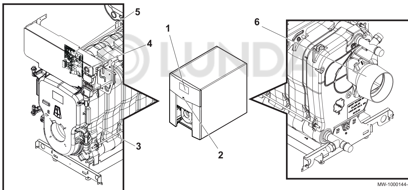
Рис.2 Основные компоненты
