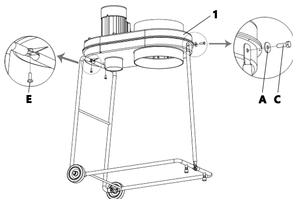
Рисунок 5. Установка корпуса
