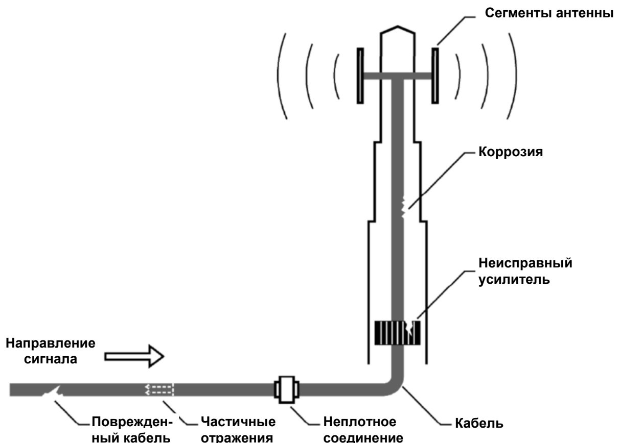
Рисунок 8.3 – Типичные дефекты передающего тракта
