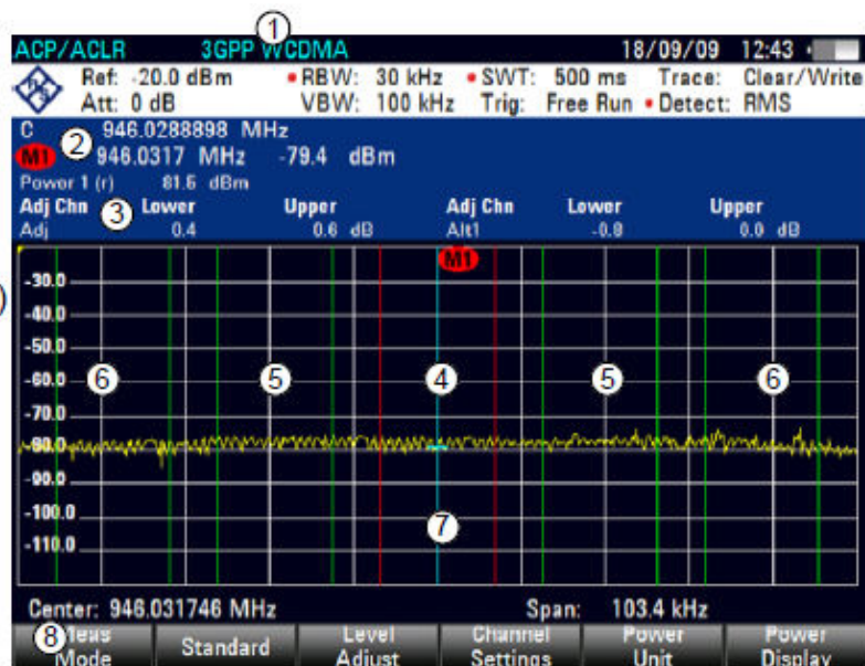
Рисунок 8.17 – Вид экрана при измерении мощности в канале
