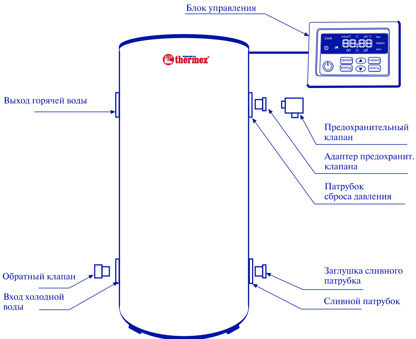
Рис. 3. Схема подключений.
