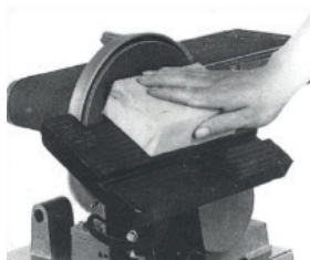
Рис. 21. Поворотное шлифование в диапазоне от 0° до 60° слева направо
