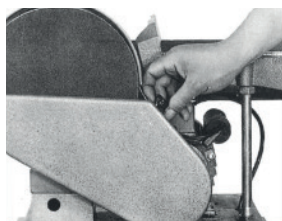
Рис. 8. Замена наждачной бумаги и клиновидного приводного ремня
