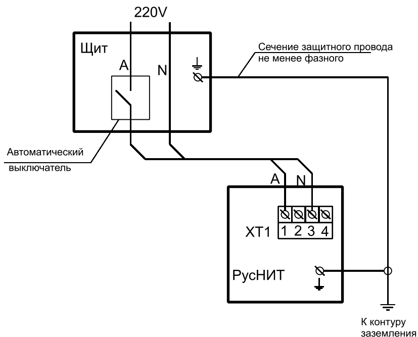
Рис.3. Схема подключения РучНИТ-203,204.
