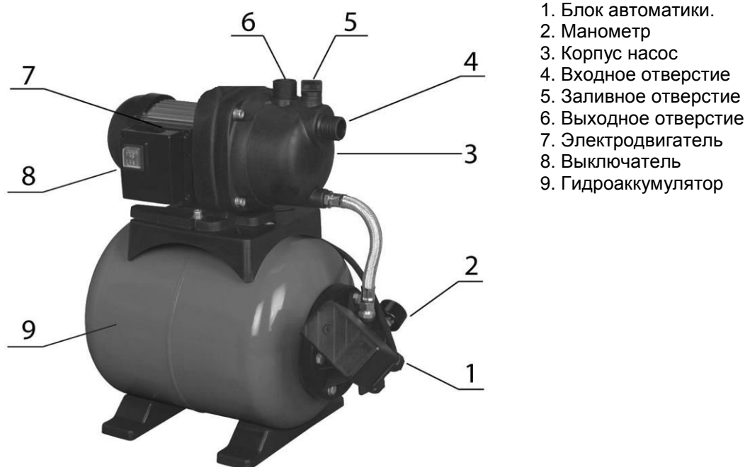
Рис.1 Модели Automatico 601, 801, 1000 Inox
