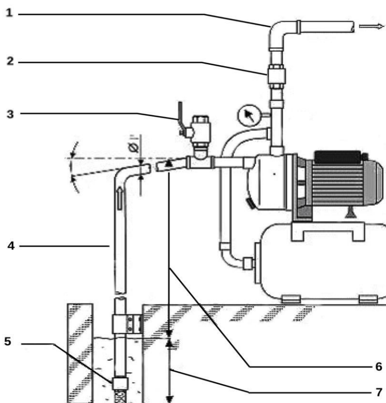
Схема стационарного монтажа насосной станции.
