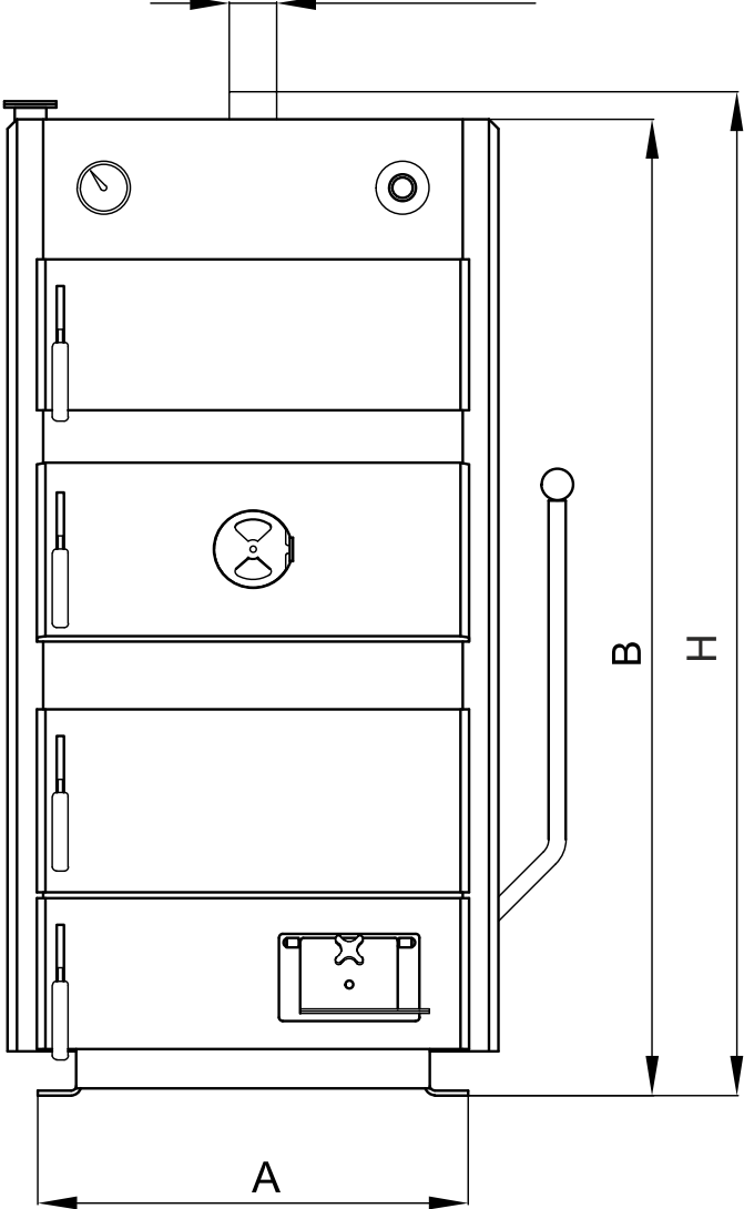
Рисунок 7.2.1 Размеры котла
