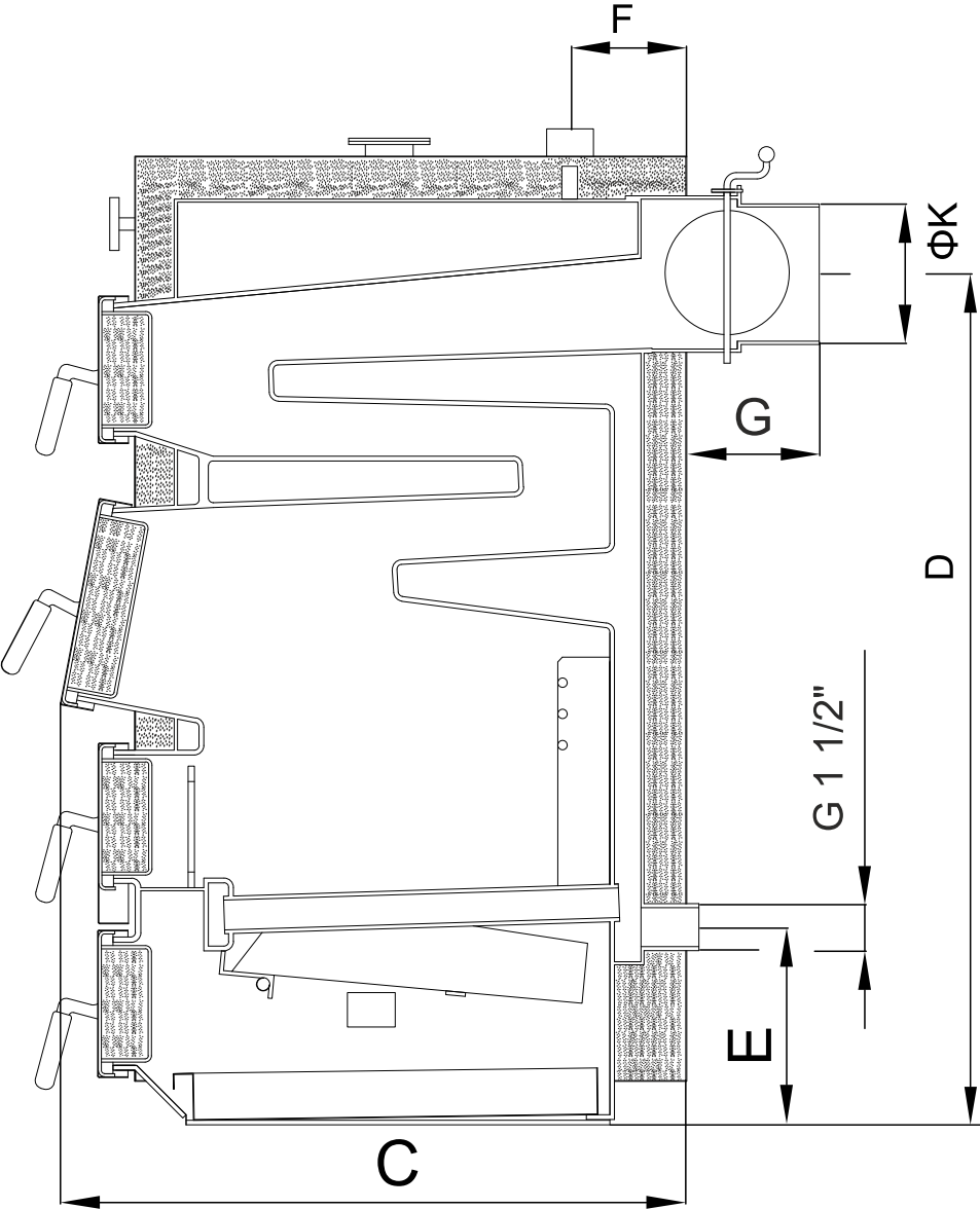
Рисунок 7.2.1 Размеры котла
