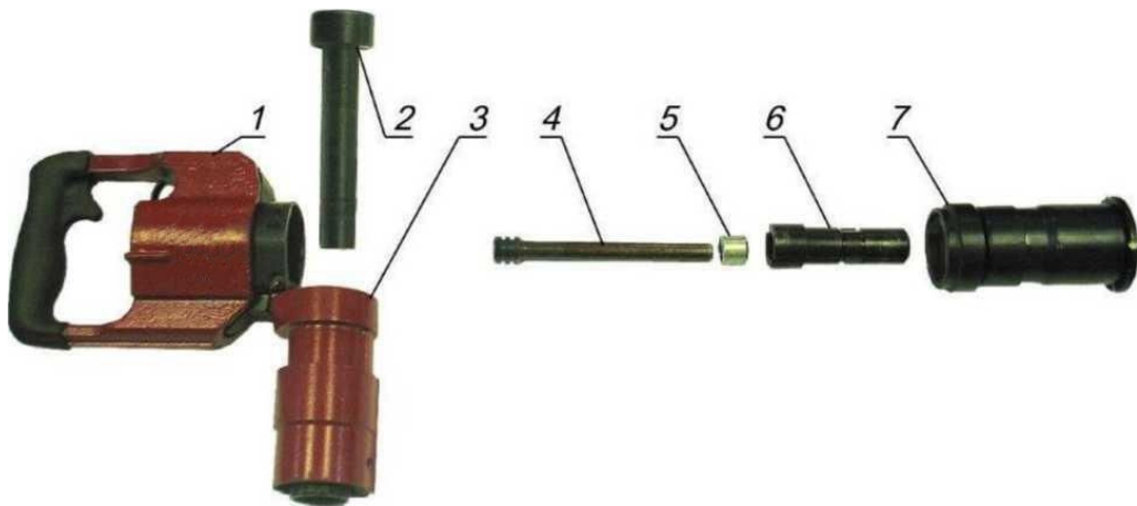
Рисунок 2 - Основные составные части пистолета
