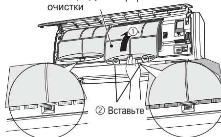
Лицевая панель
