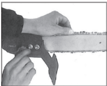
12. Отрегулируйте натяжение цепи.
