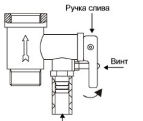
Отверстие сброса давления рис. 3
