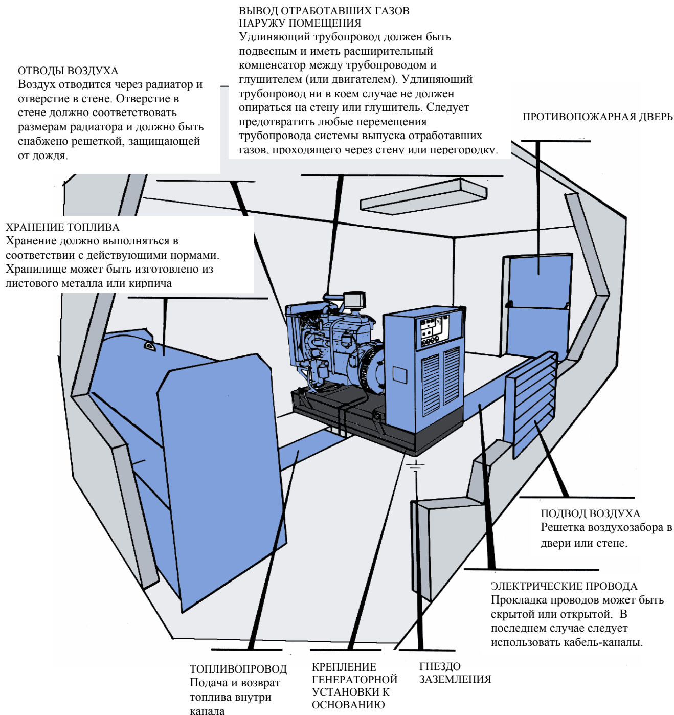
Рисунок 2.6: Пример помещения для генераторной установки
