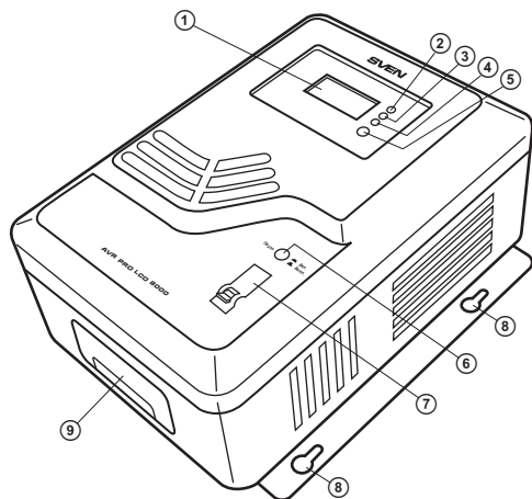
Мал. 1. Лицьова панель
