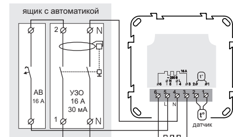
Схема 2. Подключение автоматического выключателя и УЗО
