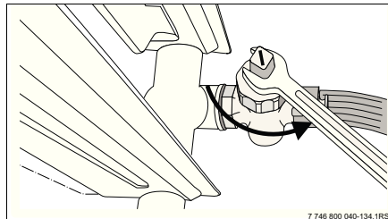
Рис 11 Слив воды из отопительной системы
