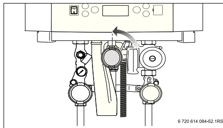
Рис 9 Закройте газовый кран
