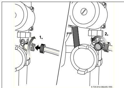
Рис 4 Подсоединение шланга
