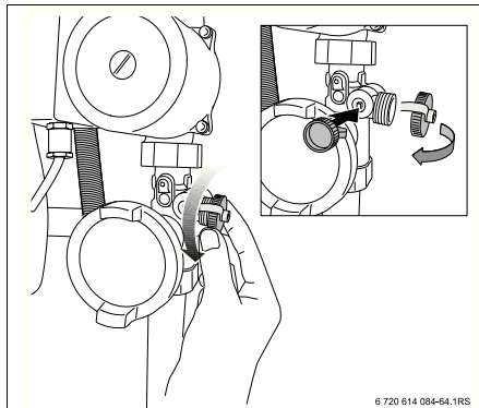
Рис 3 Крышка крана заполнения и слива
