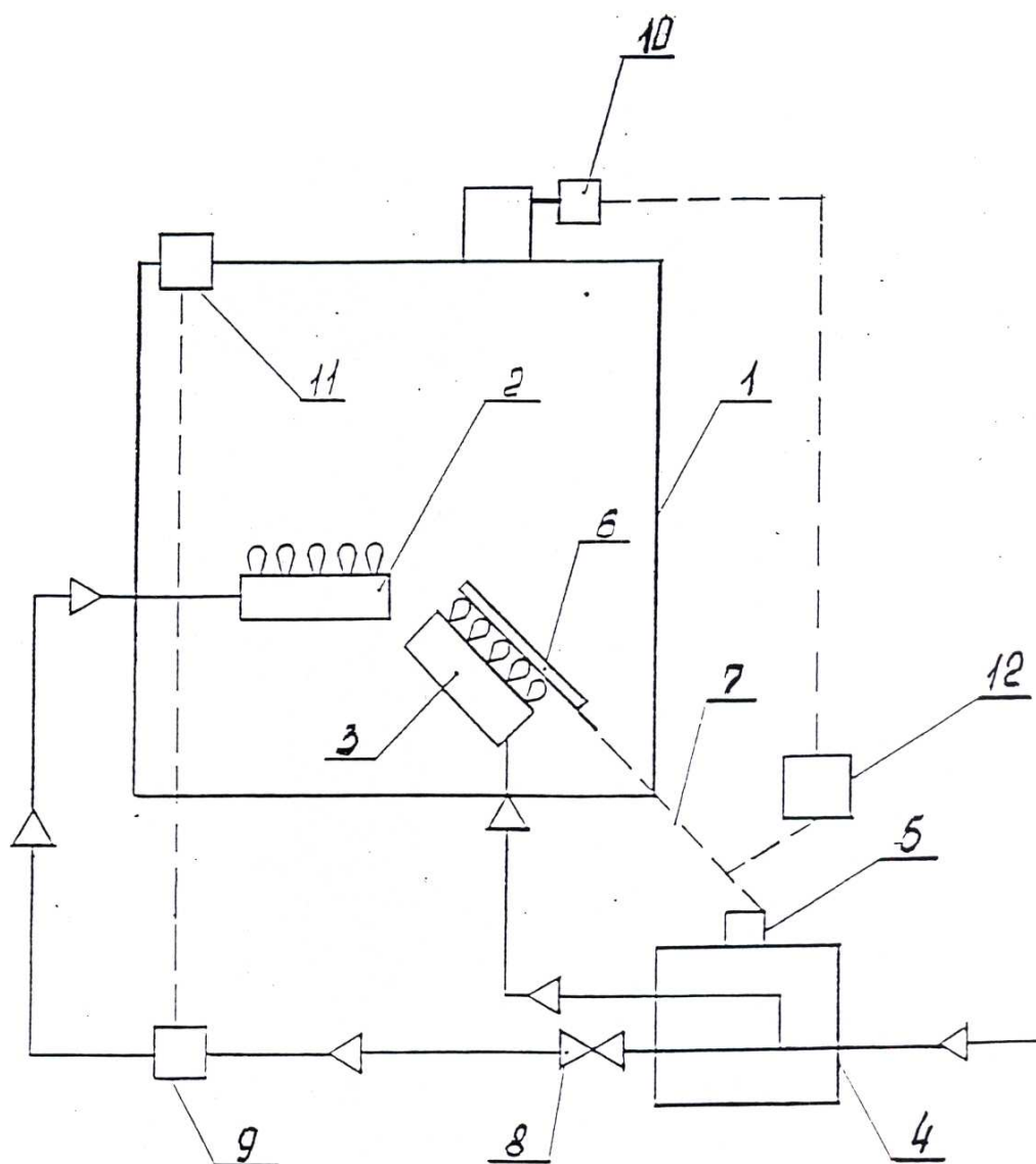
Рис. 4. Принципиальная схема
