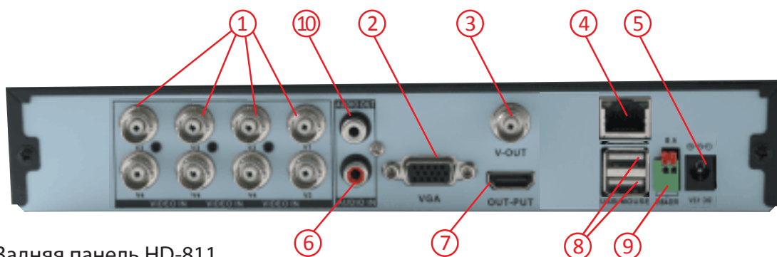
Задняя панель HD-811
