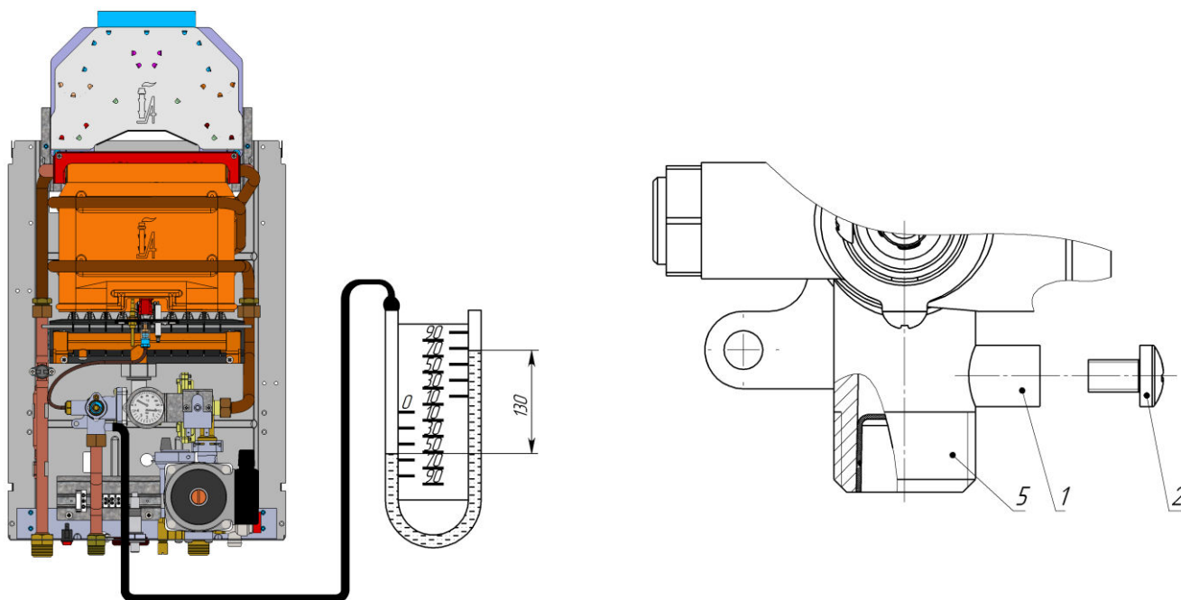
1 – патрубок замера давления газа; 2 – винт с уплотнением; 5 – входной патрубок газового узла.
