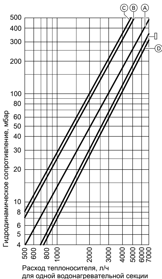
Гидродинамическое сопротивление на стороне греющего контура
