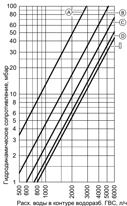
Гидродинамическое сопротивление на стороне контура водоразбора ГВС
