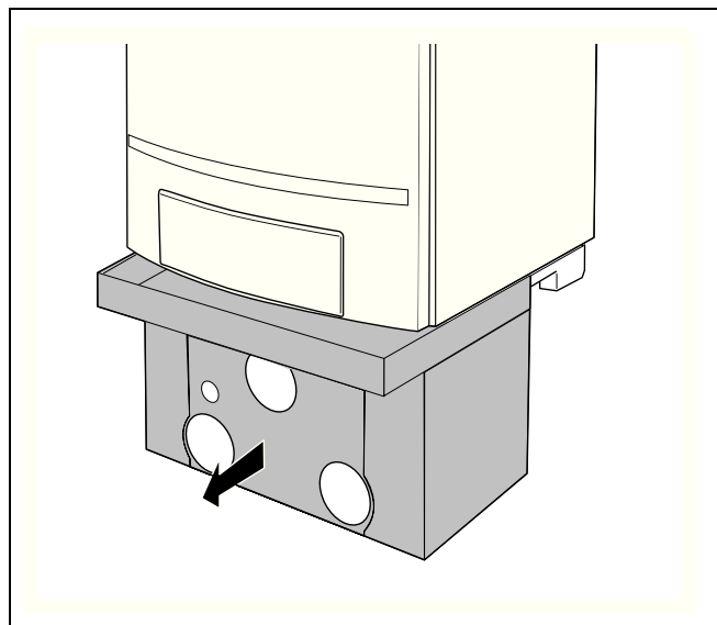
Рис. 8 Снятие нижнего кожуха
