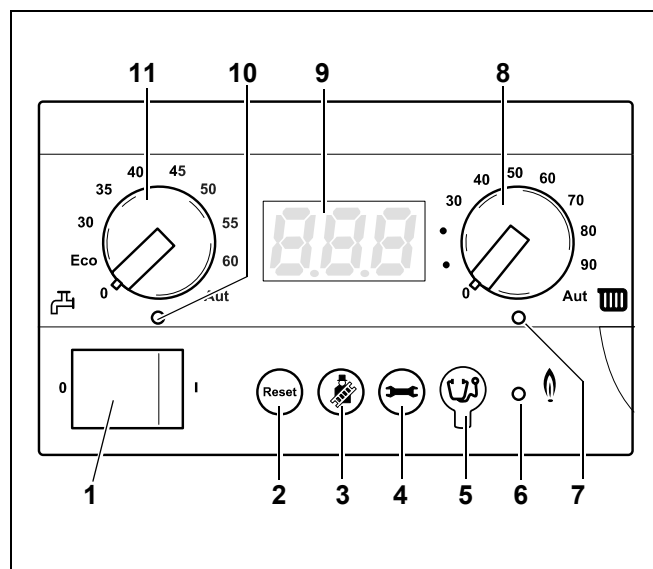
Рис.7 Главный регулятор BC10
