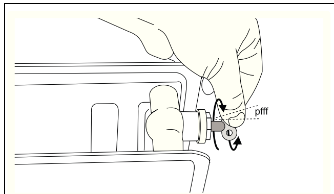
Рис. 15 Удаление воздуха из отопительного прибора
