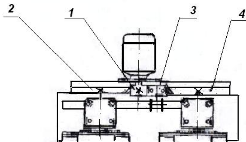
Рисунок 2 - Схема кинематическая
