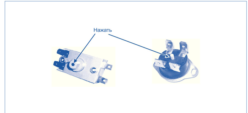
Рис. 2. Схема расположения кнопки термовыключателя.
