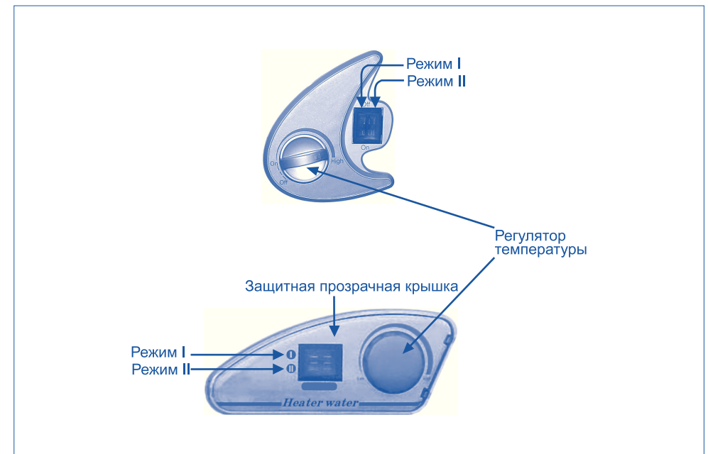
Рис. 3. Механическая панель управления.
