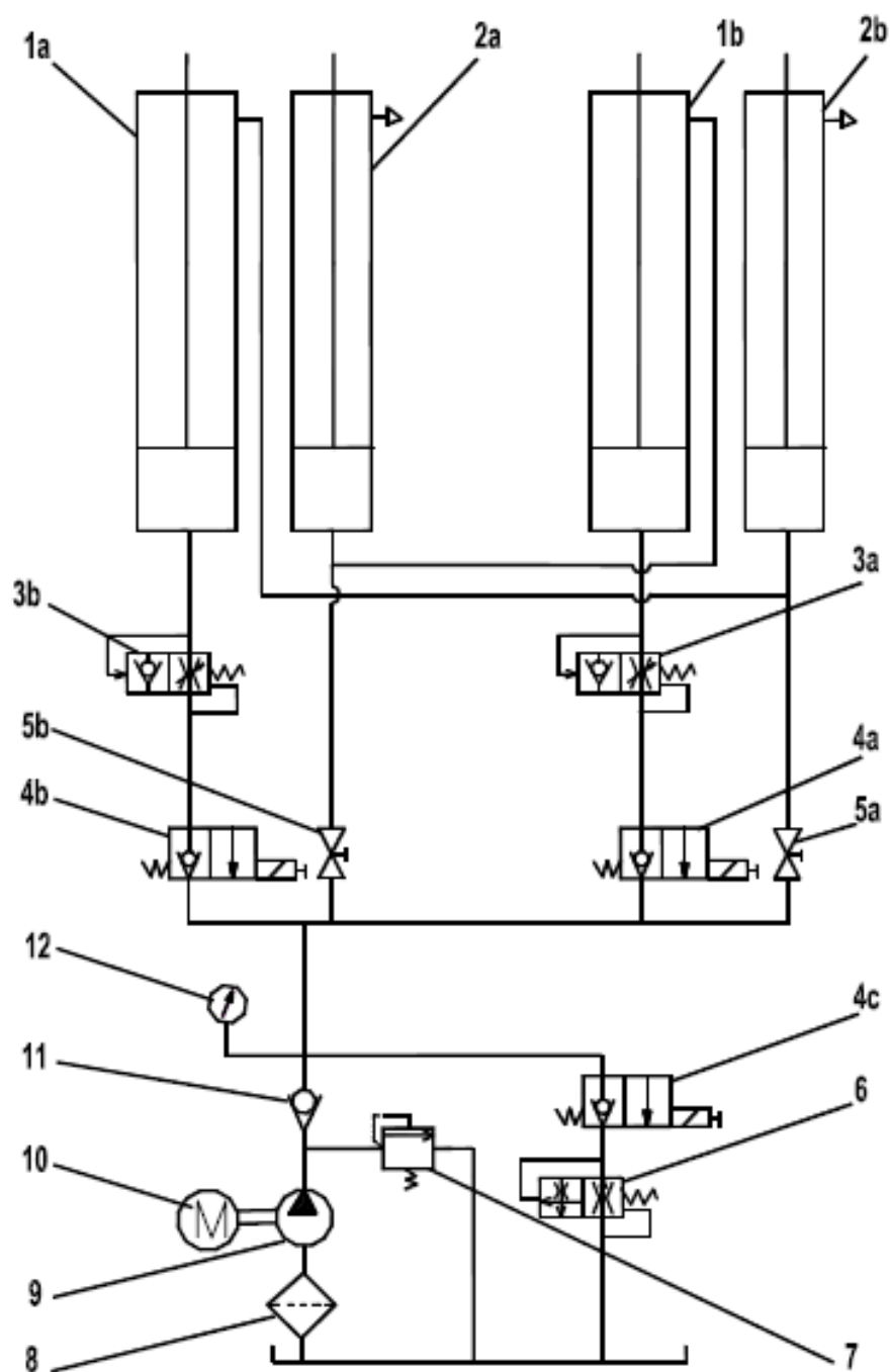
Рис.4 Гидросистема
