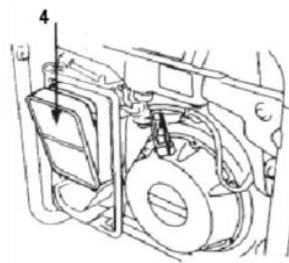
Рис.9. Снятие фильтрующего элемента
