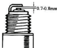
Рис. 7. Регулировка зазора в свече зажигания
