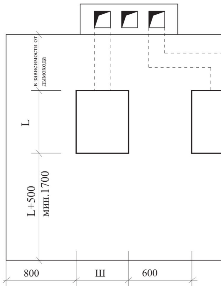
Рисунок 10 – Планировка котельной.
