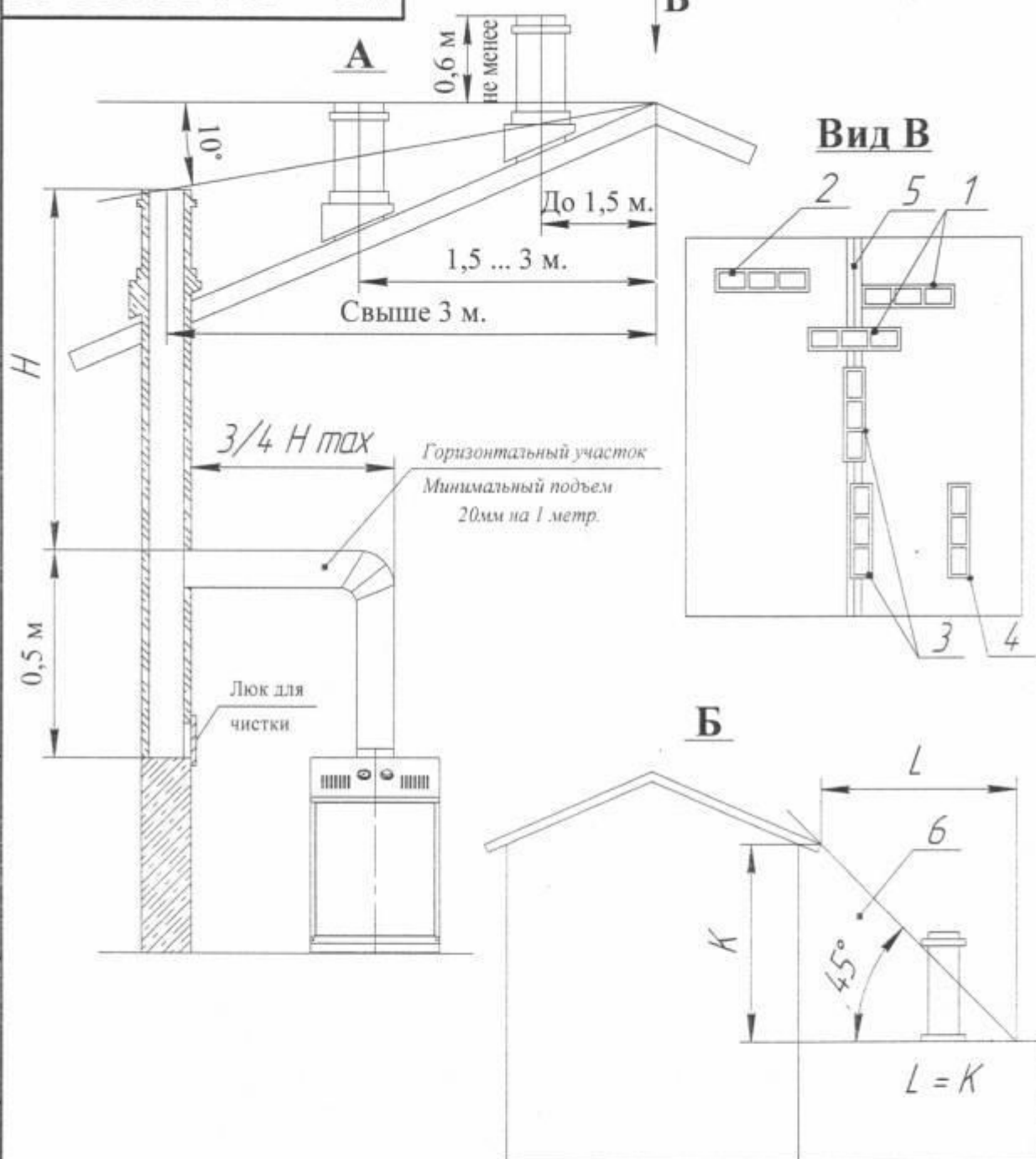
Рис. 10. Схема установки дымовой трубы.
