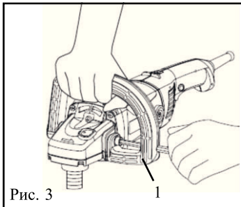
Рис. 3 1 – боковая рукоятка
