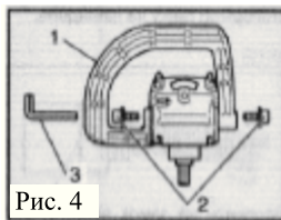
Рис. 4 1 – боковая рукоятка; 2 – болт; 3 – ключ шестигранный
