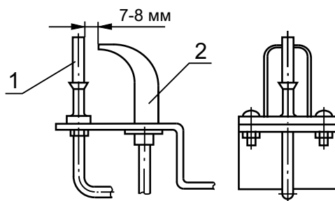
1 Термопара 2 Запальник
