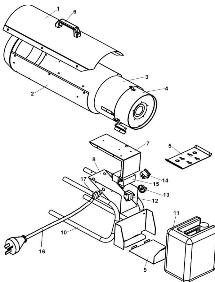
Рис. 1. Общий вид тепловой пушки.
