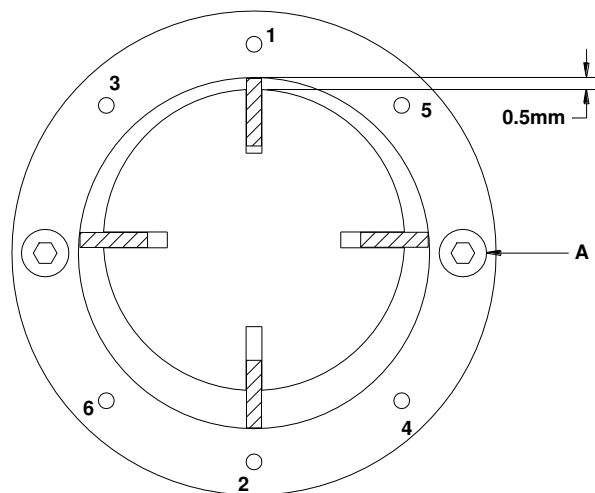
Рис.3. регулировка зазора между ротором и кольцом (компрессора).
