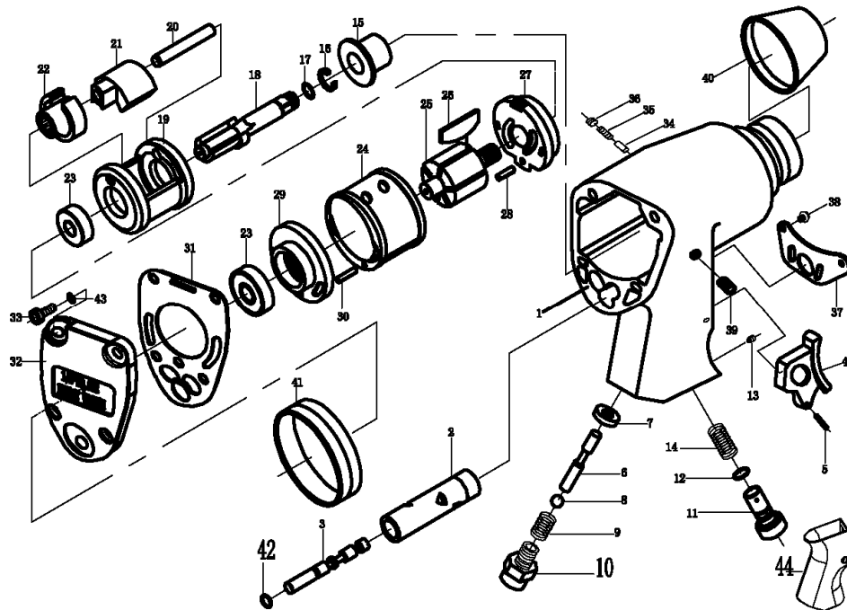
Рис.2. Схема устройства и сборки гайковерта ручного пневматического MFV 012/244-1
