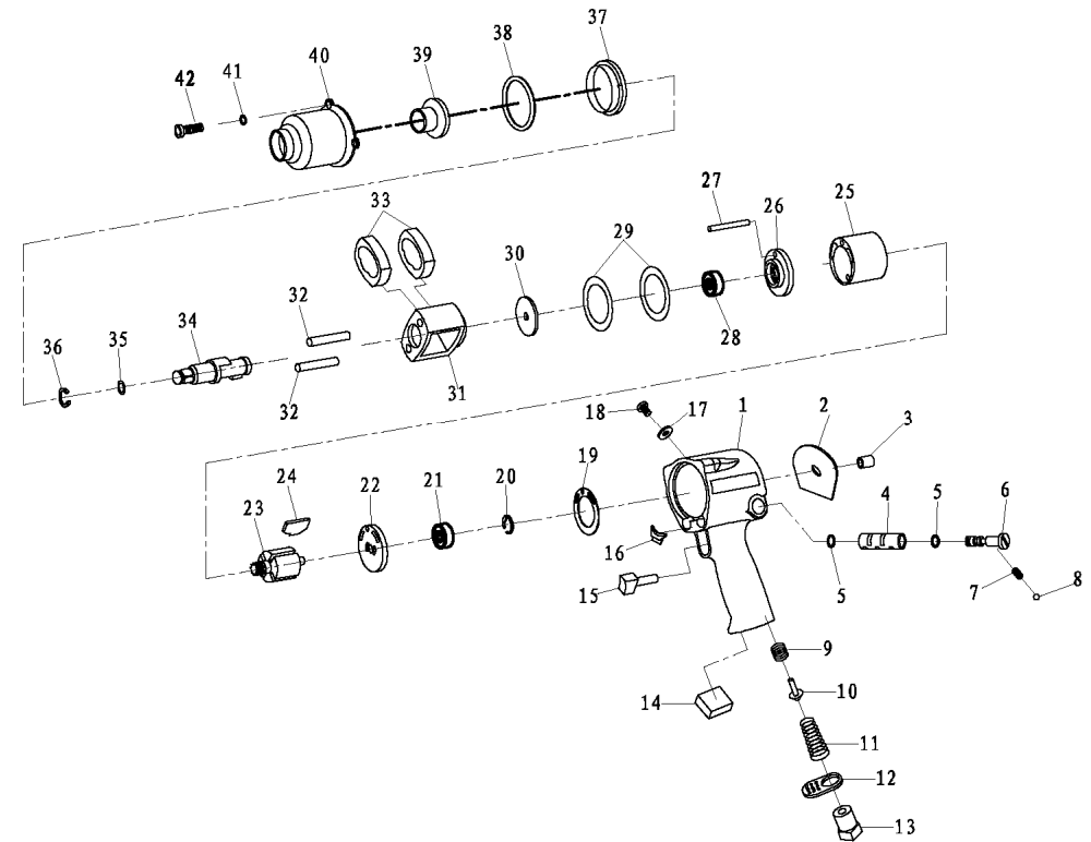
Рис.2а. Схема устройства и сборки гайковерта ручного пневматического MFV 016/610-1.
