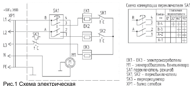
Рис.1 Схема электрическая
