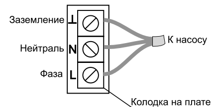
Рис.5 Подключение циркуляционного насоса
