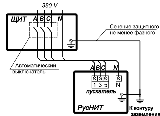
Рис.6 Схема подключения к трехфазной сети
