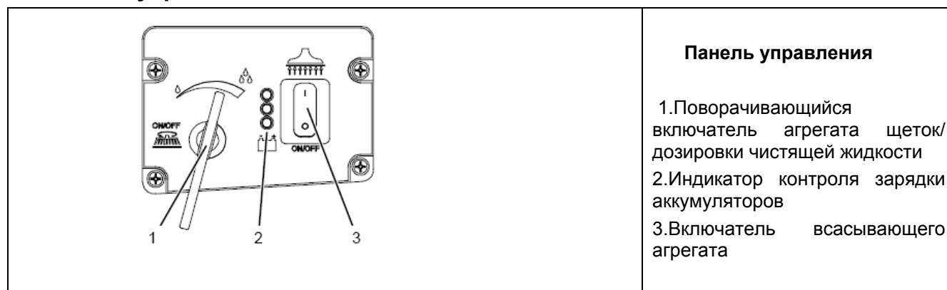
Рис.2 Панель управления
