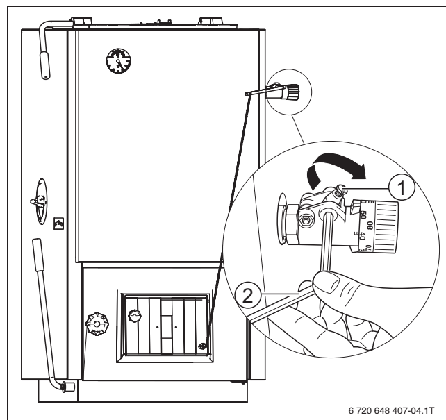
Рис. 7 Монтаж регулятора горения
