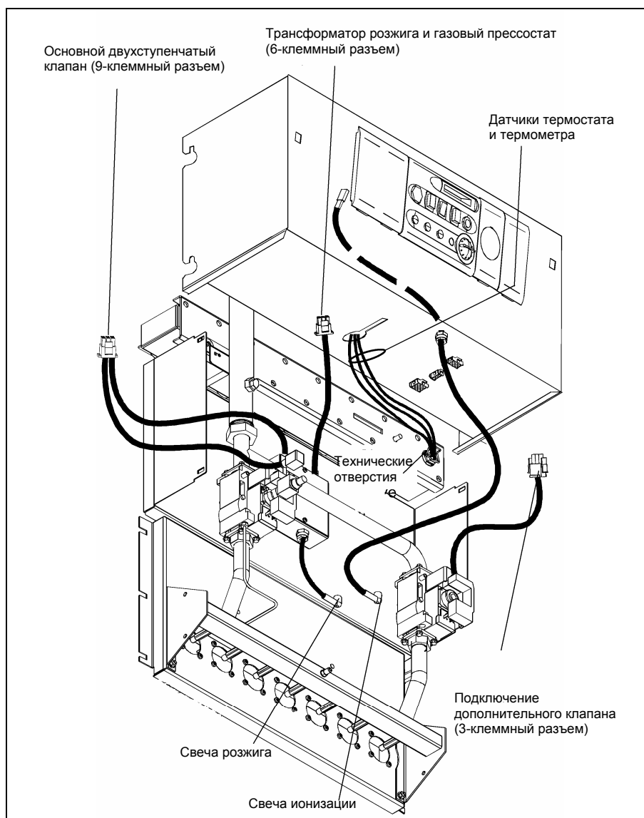
Технические отверстия котла без датчика регулировок
