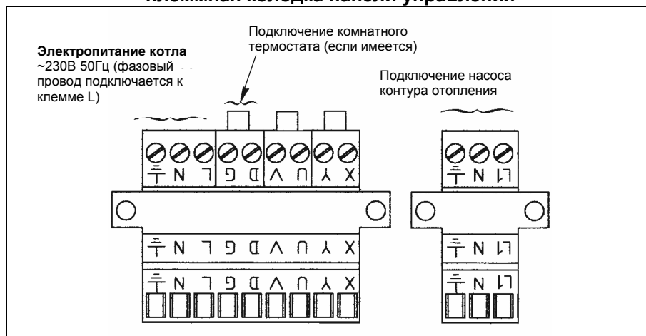
Клеммная колодка панели управления
