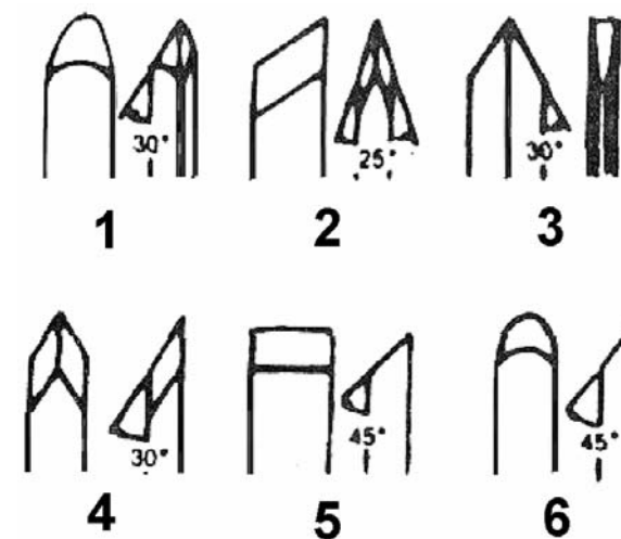
Рис. 15 – Шесть наиболее распространенных типов резцов
