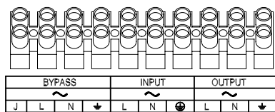
VGД 4/5/6K TB
