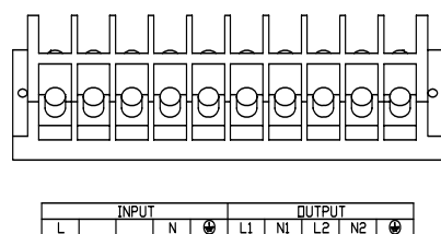
VGД 15/20K-ISO TB
