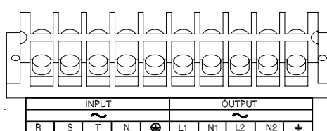
VGД 8/10/12K-ISO-3 фазы TB
