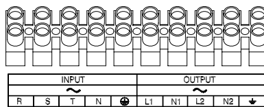
VGД 8/10/12K-3 фазы TB
