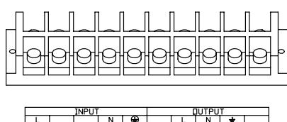
VGД 15/20K TB
