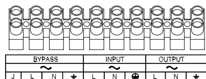
VGД 8/10/12K TB
