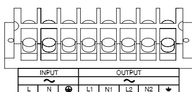
VGД 4/5/6/8/10/12K-ISO TB
