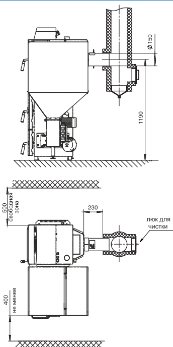
Рис.7 Схема установки котла
